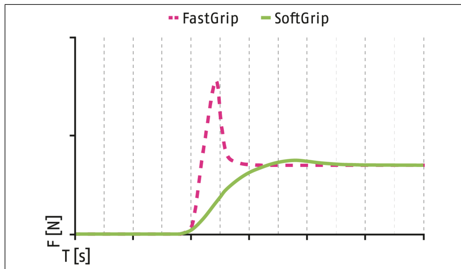
Kraftverlauf bei FastGrip und SoftGrip
